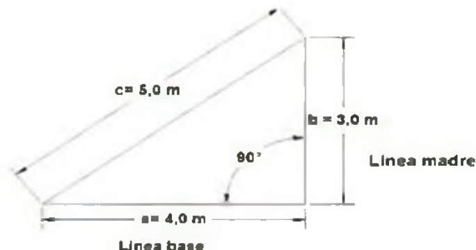
Fig. 37. Uso del teorema de Pitágoras 3, 4 y 5 para trazar la línea madre
