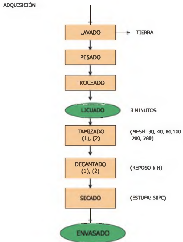
Figura 4.8. Diagrama del proceso para la obtención de almidón de RTAs.
