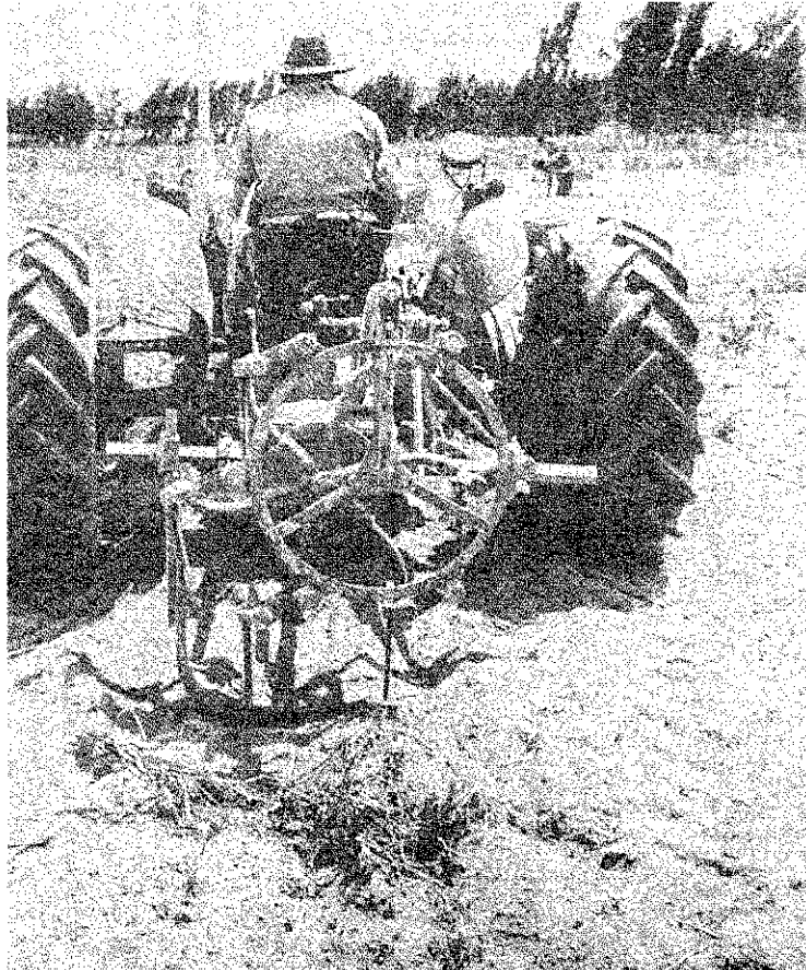
FOTO 1.- Cavadora de molinete.
